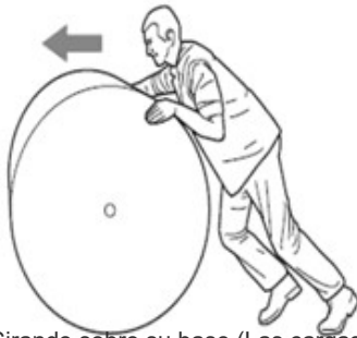
Girando sobre su base (Las cargas se mueven girando/rodando a lo largo de los bordes de su base):
